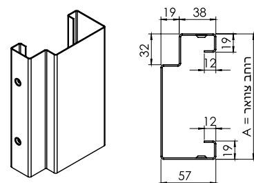
משקוף חובק גבס
