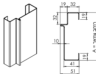
משקוף בנייה אומניוית+ חיפוי אומניוית
