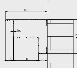
משקוף קו אפס עם צירים נסתרים
