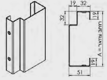
משקוף חובק גבס
