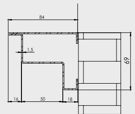
משקוף קו אפס
