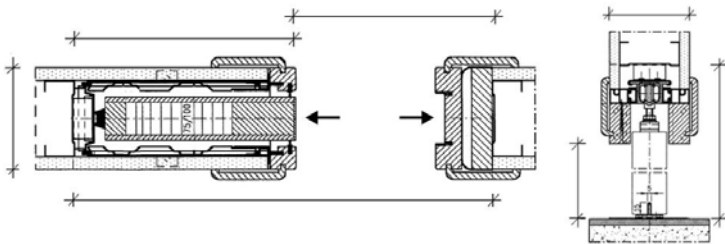
מפרט דלתות הזזה לתוך כיס
