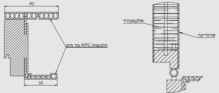
משקוף עץ מפולח גושני הלבשות WPC
