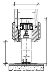
חתך כיס
