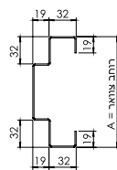
משקוף דגם 800 לביטון עם פלס כפול
