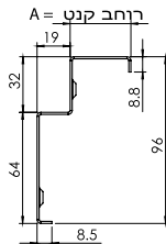
משקוף כיסוי להתקנה על משקוף קיים
