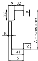
משקוף בנייה אומניות לביטון כולל חיפוי אומניות
