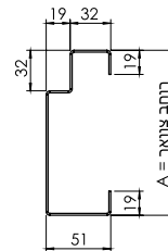
משקוף דגם c לביטון
