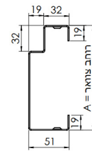
משקוף חובק גבס
