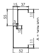
משקוף מוסדי דגם c לביטון/חובק לדלתות פורמייקה עם חריץ לאטם
