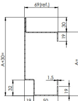
משקוף הדס לביטון כולל שן לחיפוי קיר
