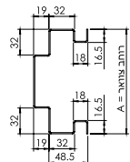
משקוף דגם 800 מתועש לביטון עם שן טיח
