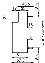
משקוף דגם c מתועש לביטון כולל שן לטיח
