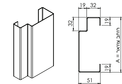
משקוף דגם C (ניתן להזמין עם/בלי הלבשות קליק)
