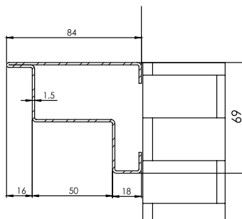
משקוף קו אפס
