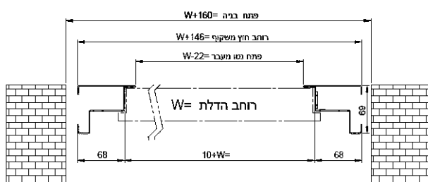
משקוף קו אפס עם צירים נסתרים
