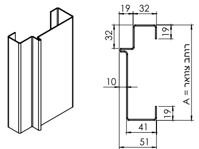
משקוף בנייה אומניוורסל חיפוי אומניוורסל
