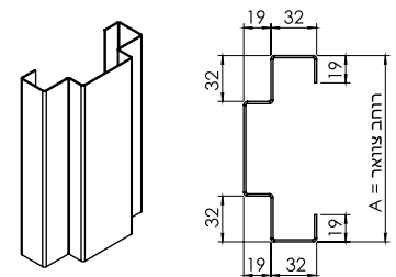
דגם 800
