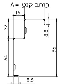
משקוף כיסוי
