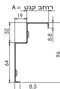
משקוף כיסוי
