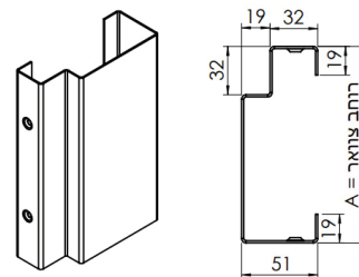
משקוף חובק גבס / דגם c
