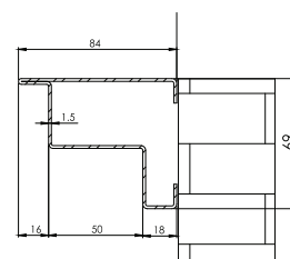
משקוף קו אפס / קו אפס עם צירים נסתרים
