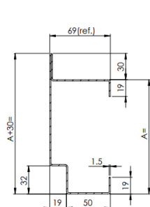
משקוף הדס
