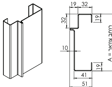
משקוף בנייה אומנויות
