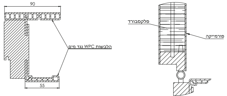
משקוף עץ מכולח גושני הלבשות WPC
